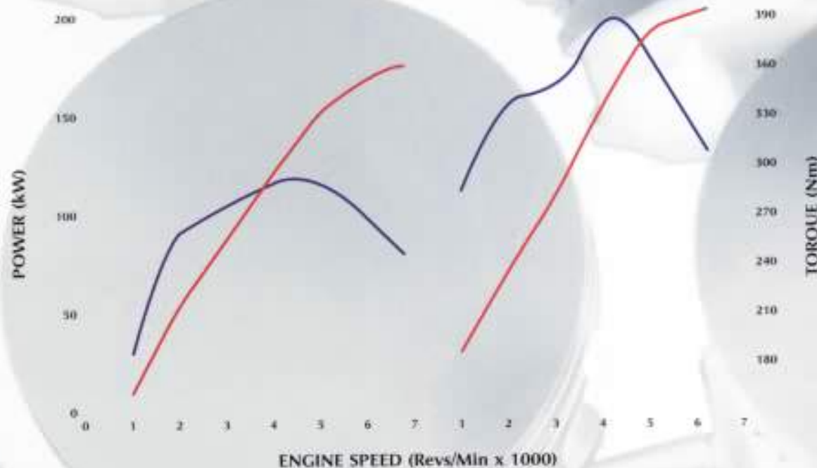
3.0 LITRE AJ-V6
